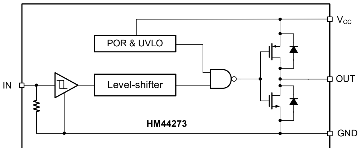
图 9-1 HM44273 功能框图
