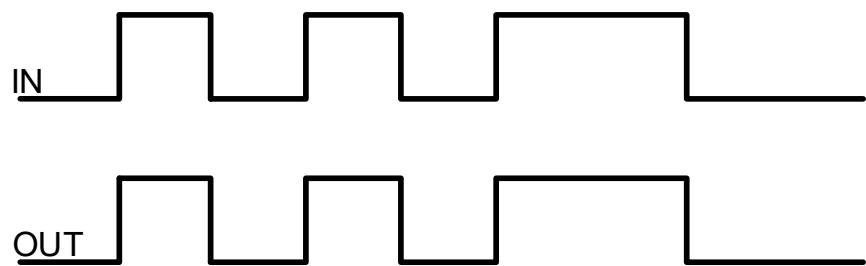
图 8-1 输入输出波形图
