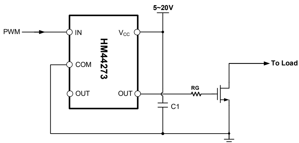
图 9-2 HM44273 典型应用电路图
